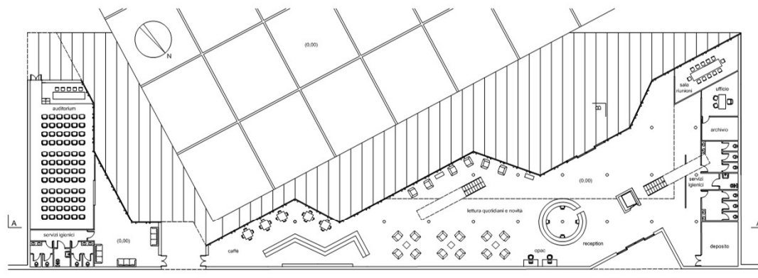
PIANTA I LIVELLO
