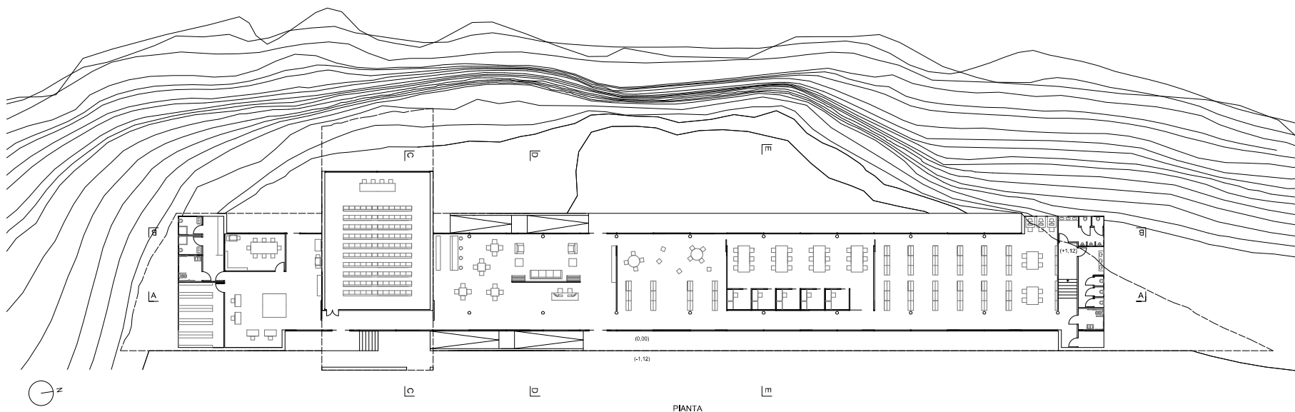
PIANTA
